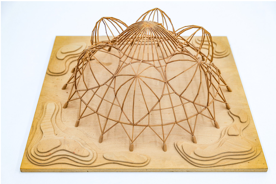
Abbildung 3: Räumliche Stabwerkkonstruktion aus dem Unterricht von Kälberer
